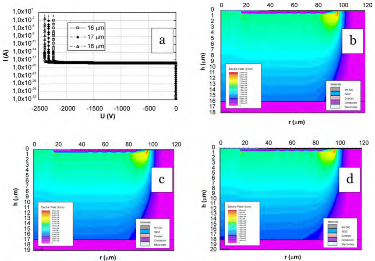
Рис. 2. а) рассчитанная обратная вольт-амперная характеристика диода Шоттки с концентрацией эпитаксиального слоя 4Н-SiC 3,75 \times 10^{15} \text{ см}^{-3} и различной толщиной эпитаксиального 4Н-SiC слоя – 16, 17 и 18 мкм; б) распределение электрического поля диода Шоттки с толщиной эпитаксиального 4Н-SiC слоя 16 мкм; в) распределение электрического поля диода Шоттки с толщиной эпитаксиального 4Н-SiC слоя 17 мкм; д) распределение электрического поля диода Шоттки с толщиной эпитаксиального 4Н-SiC слоя 18
