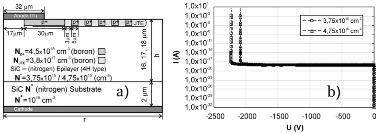
Рис. 1. а) структура карбидокремниевого диода Шоттки для расчета; б) рассчитанная обратная вольт-амперная характеристика диода Шоттки типа 4Н-SiC при различных концентрациях эпитаксиального слоя 4Н-SiC – 3,75 \times 10^{15} \text{ см}^{-3} и 4,75 \times 10^{15} \text{ см}^{-3}
