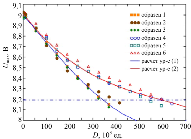
Рис. 3. Экспериментальные и расчетные зависимости выходного напряжения U_{\text{вых}} линейного стабилизатора напряжения ИС-ЛС-9В от уровня поглощенной дозы D при U_{\text{вх}} = 9,5 В и I_{\text{н}} = 1 А (режим 3, образцы 1, 2, 3) и U_{\text{вх}} = 24 В и I_{\text{н}} = 10 мА (режим 2, образцы 4, 5, 6). Точки – эксперимент, линии – расчет. Штрихпунктирная линия – граница нормы по выходному напряжению
